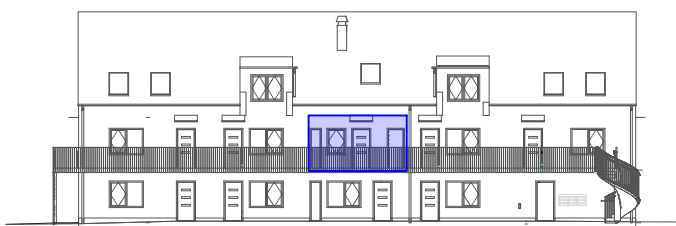
FASAD HUS 3 - NORR VÄSTRA JÄRNVÄGSGATAN 12
