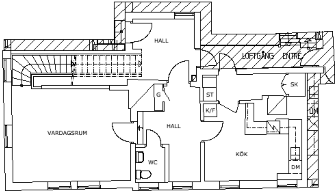
Nedre plan
