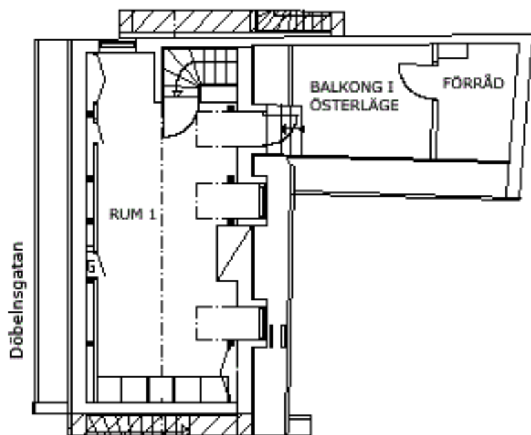
Övre plan
