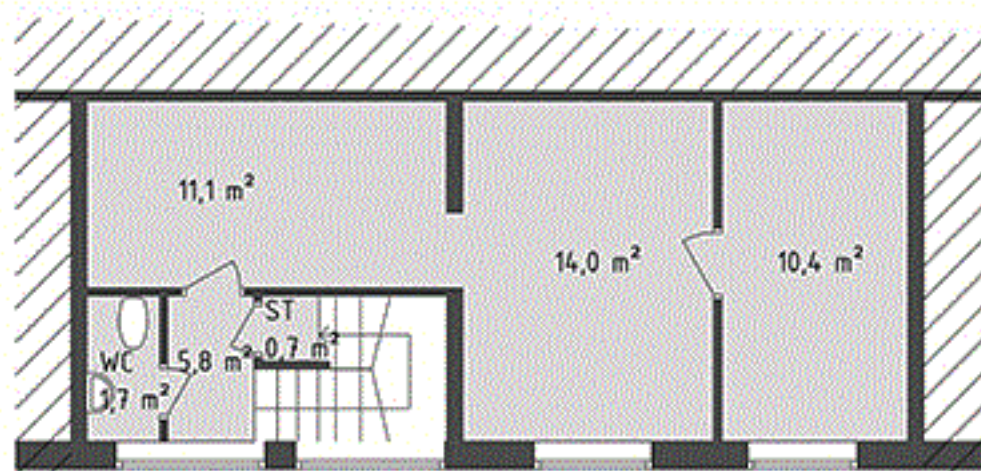
KÄLLARPLAN
